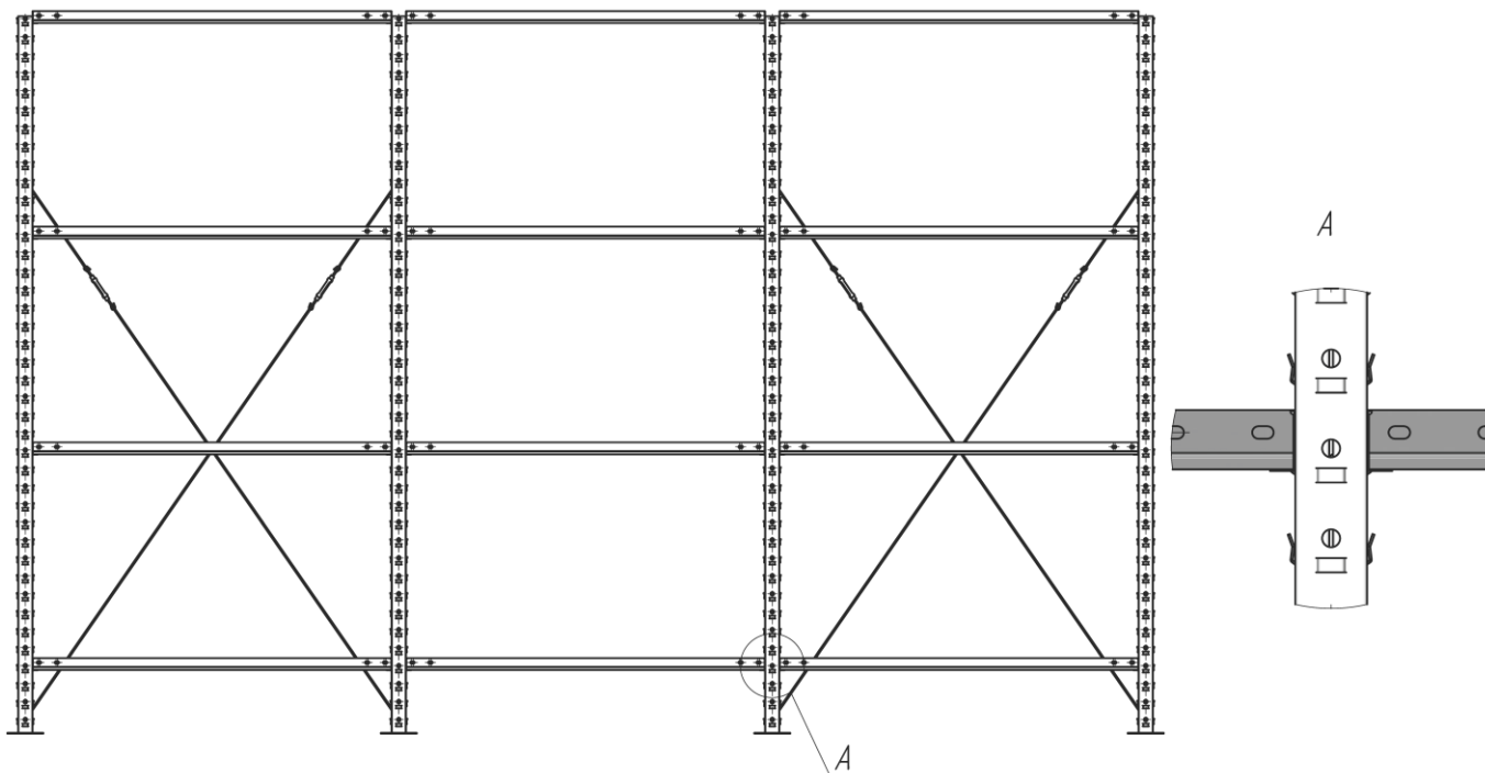
Рис. 8 – Эскиз соединения стеллажей в линейку
