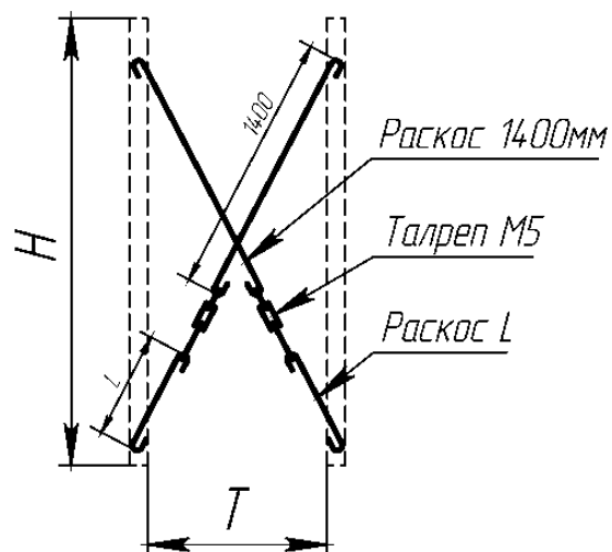
Рис. 4 – Схема сборки крестовины жесткости
