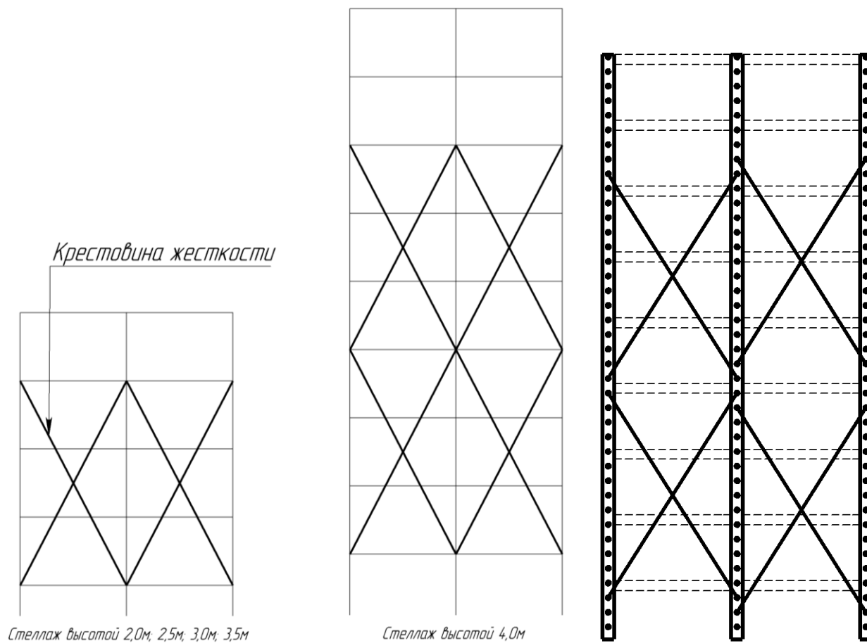
Рис. 6 – Схема распределения крестовин жесткости и их крепление на стойках
