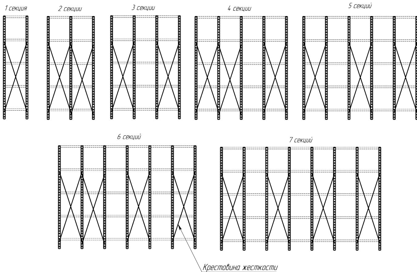
Рис. 5 – Схема установки крестовин жесткости
