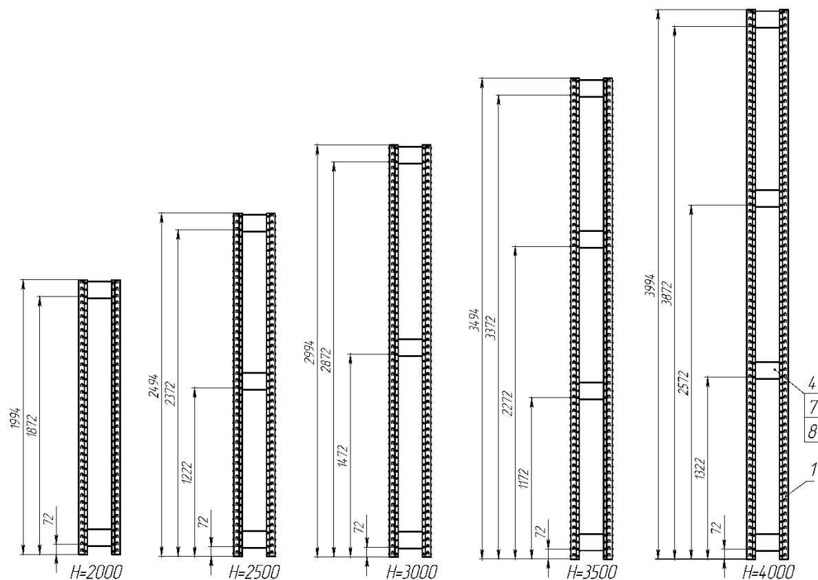
Рис. 3 – Схема установки стяжек поперечных для рам разной высоты 1 – СГ стойка; 2 – СГ подпятник; 3 – СГ стяжка поперечная; 4 – Болт М6х12; 5 – Гайка М6;
