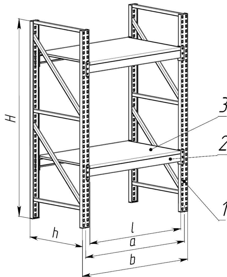
Рисунок 1 – Схема сборки секции стеллажа СГ
